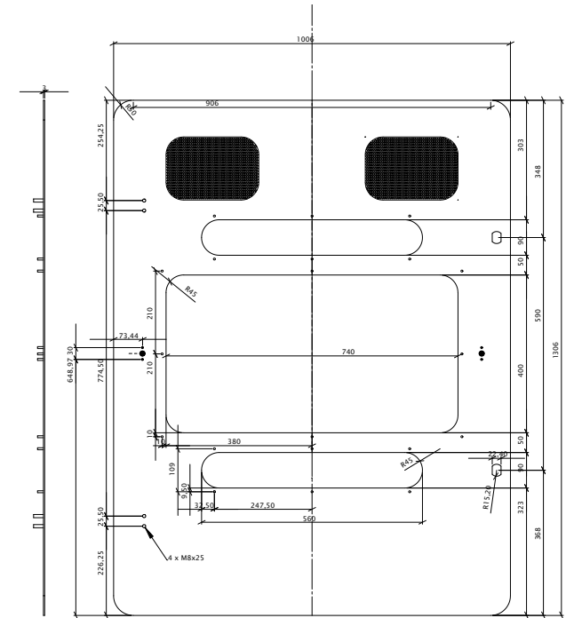
Fertigungszeichnung Interface-Element
