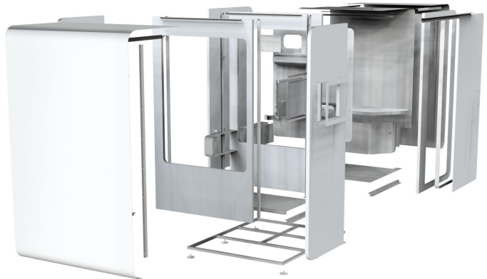
Explosionsdarstellung
